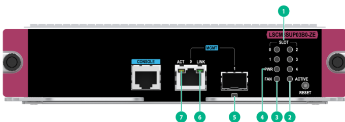
图1-3 LSCM3SUP03B0-ZE 主控板指示灯示意图
