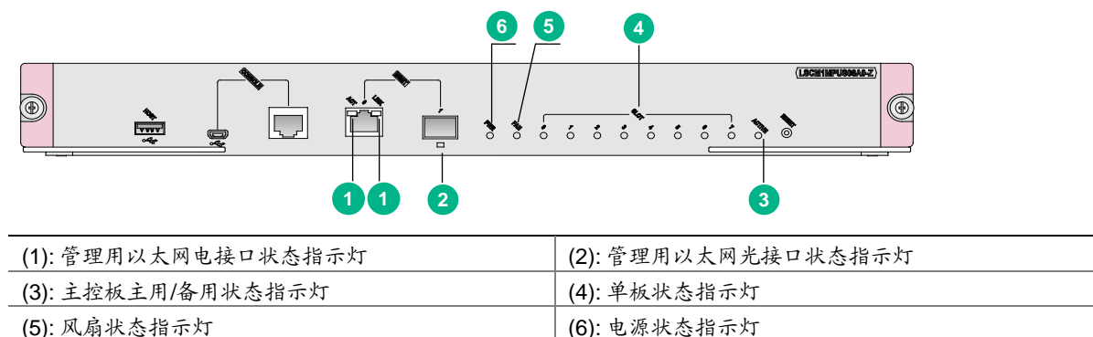
图1-4 LSCM1MPUS06A0-Z 主控板指示灯示意图
