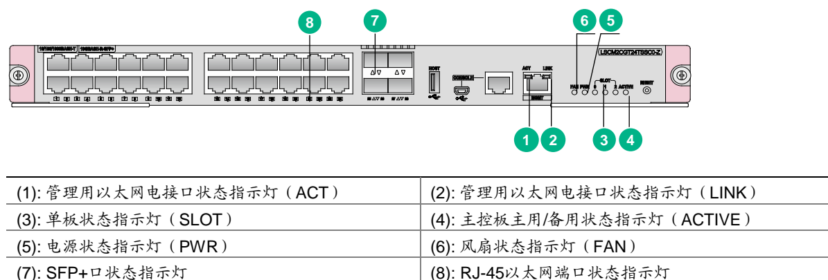
图1-5 LSCM2CGT24TSSC0-Z 主控板指示灯示意图
